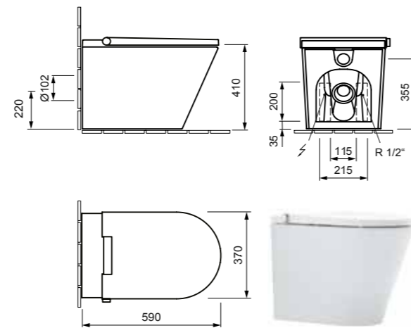
E101-0304 AXENT ONE floorstanding
