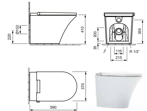
E101-0306 AXENT ONE Plus floorstanding
