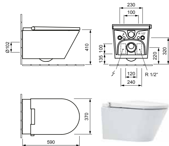
E101-0301 AXENT ONE wall-mounted
