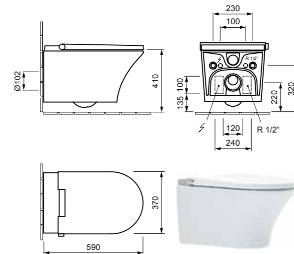
E101-0303 AXENT ONE Plus wall-mounted
